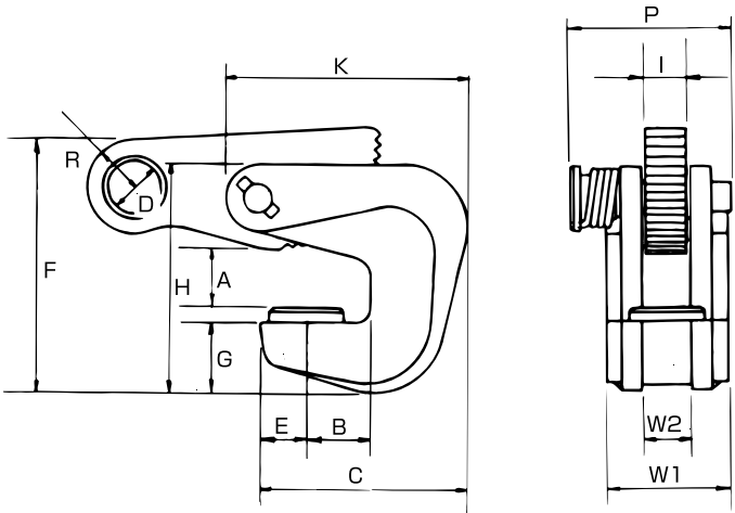
●寸法図
