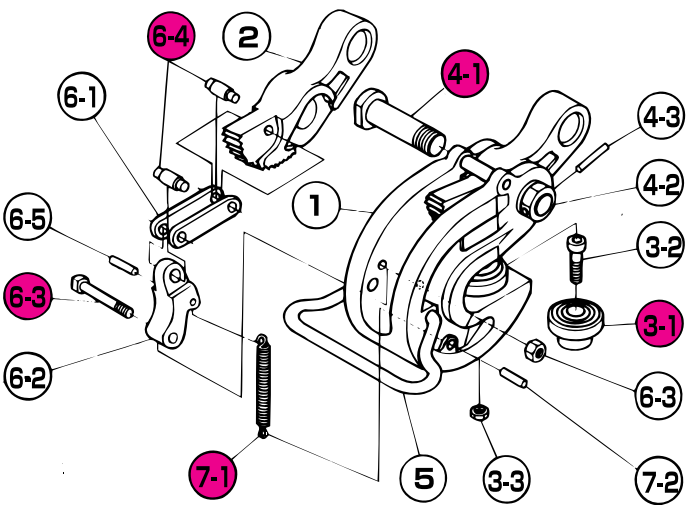
●分解構造図
