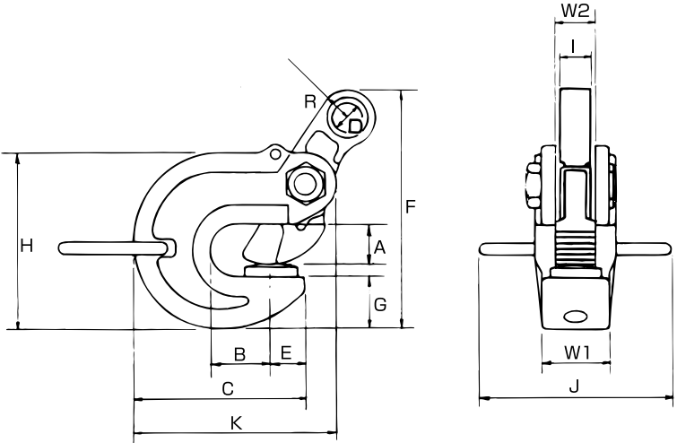
●寸法図
