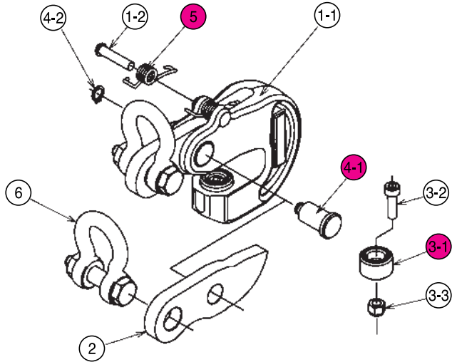
●部品名
