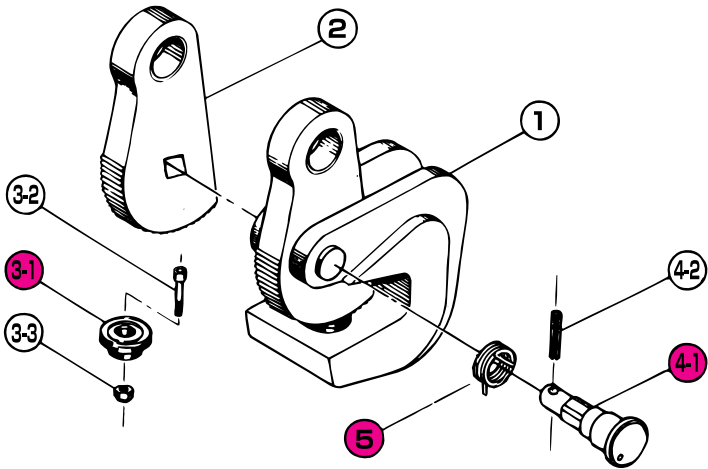
●分解構造図
