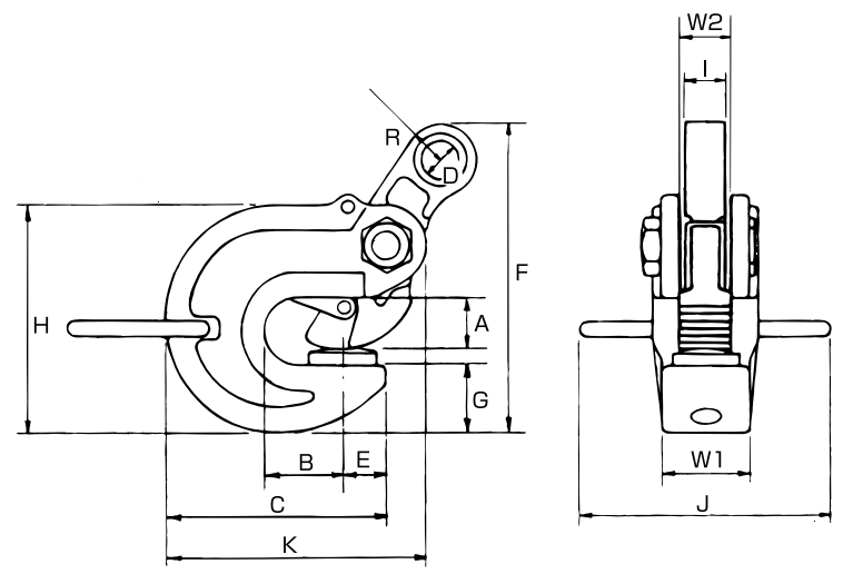
●寸法図
