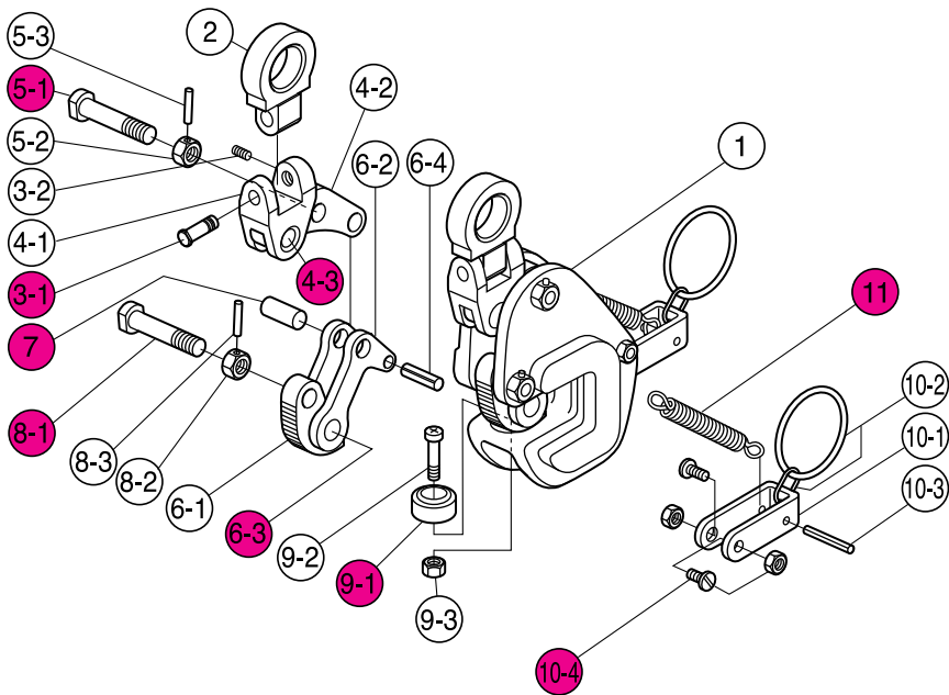
●分解構造図
