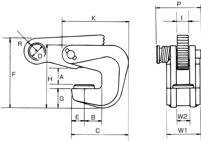
●寸法図
