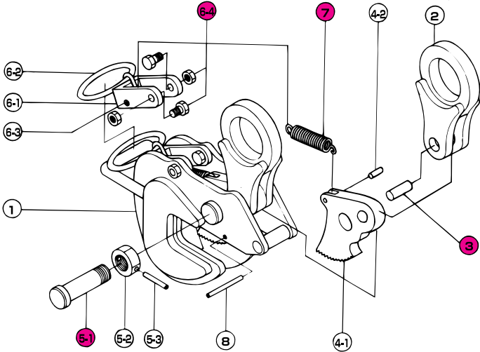
分解構造図
