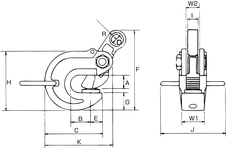
●寸法図
