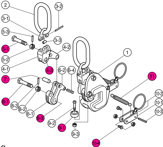
分解構造図
