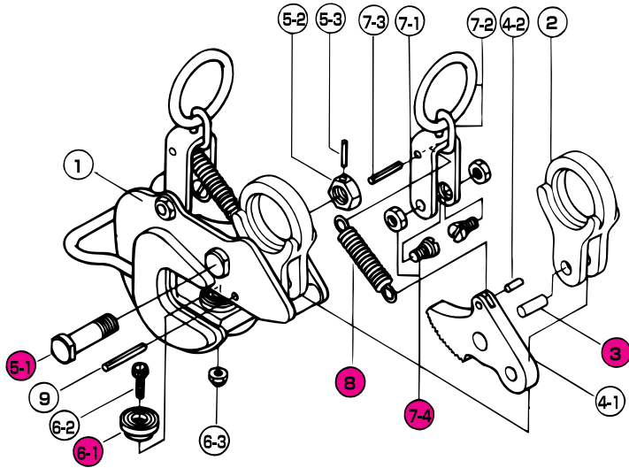
●分解構造図
