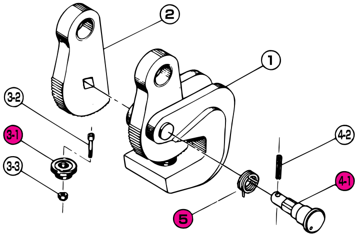
●分解構造図
