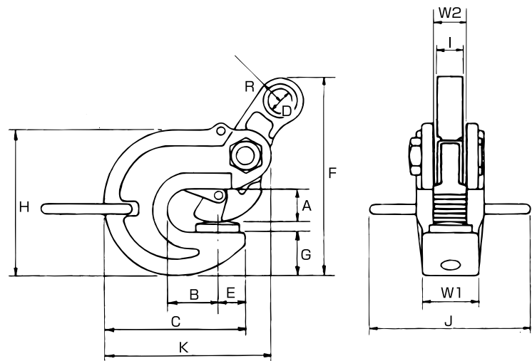
●寸法図
