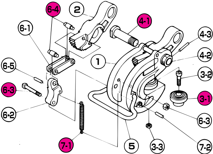
●分解構造図
