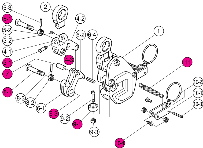
●分解構造図
