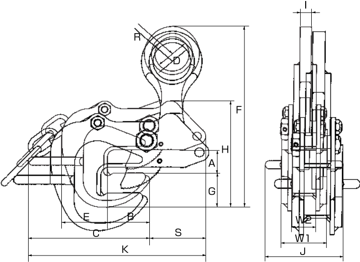
寸法図
