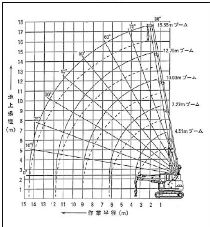
■ CK120UR-1E 作業範囲図
