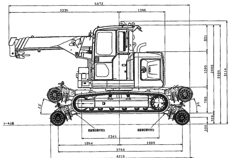
※在来線走行姿勢図
