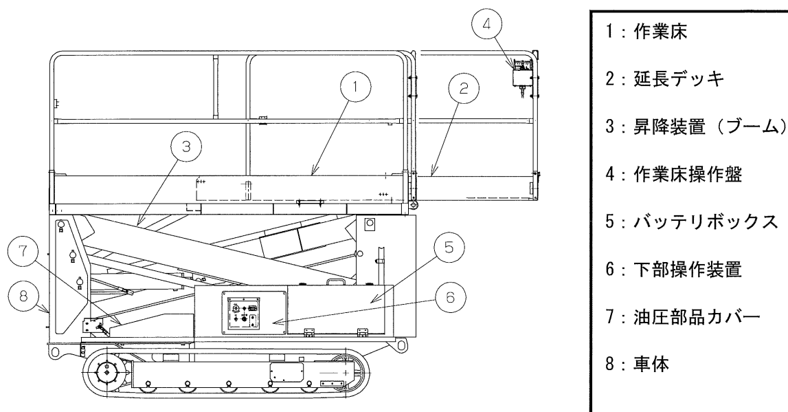
図 高所作業車の概要
