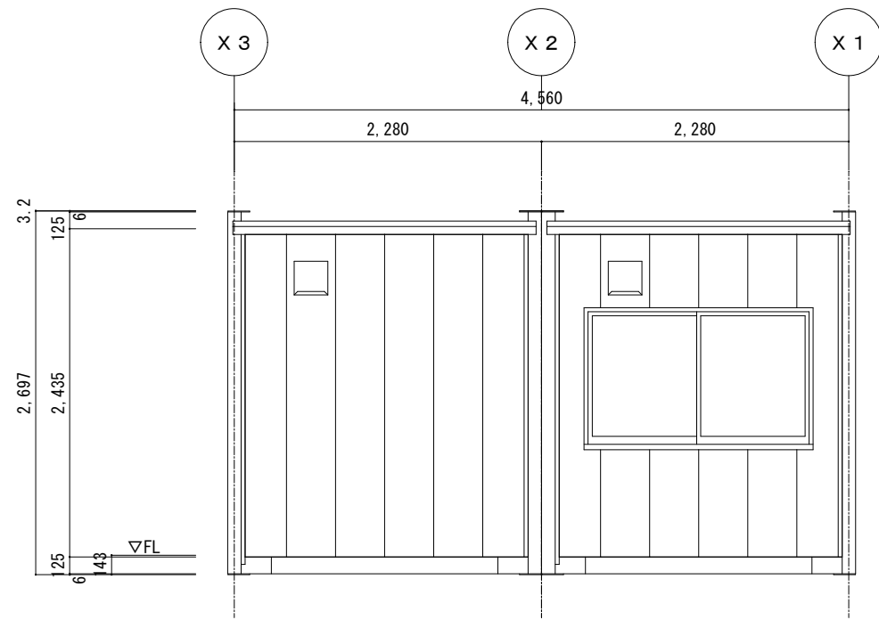
A側立面図 S = 1/50
