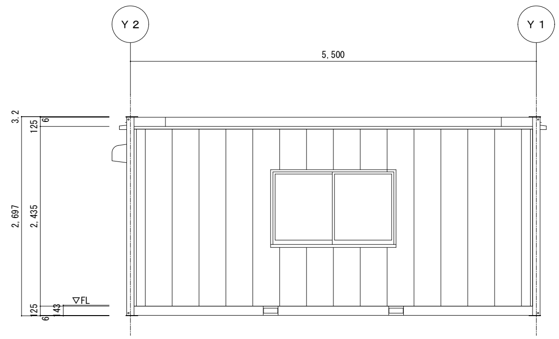
D側立面図 S = 1/50
