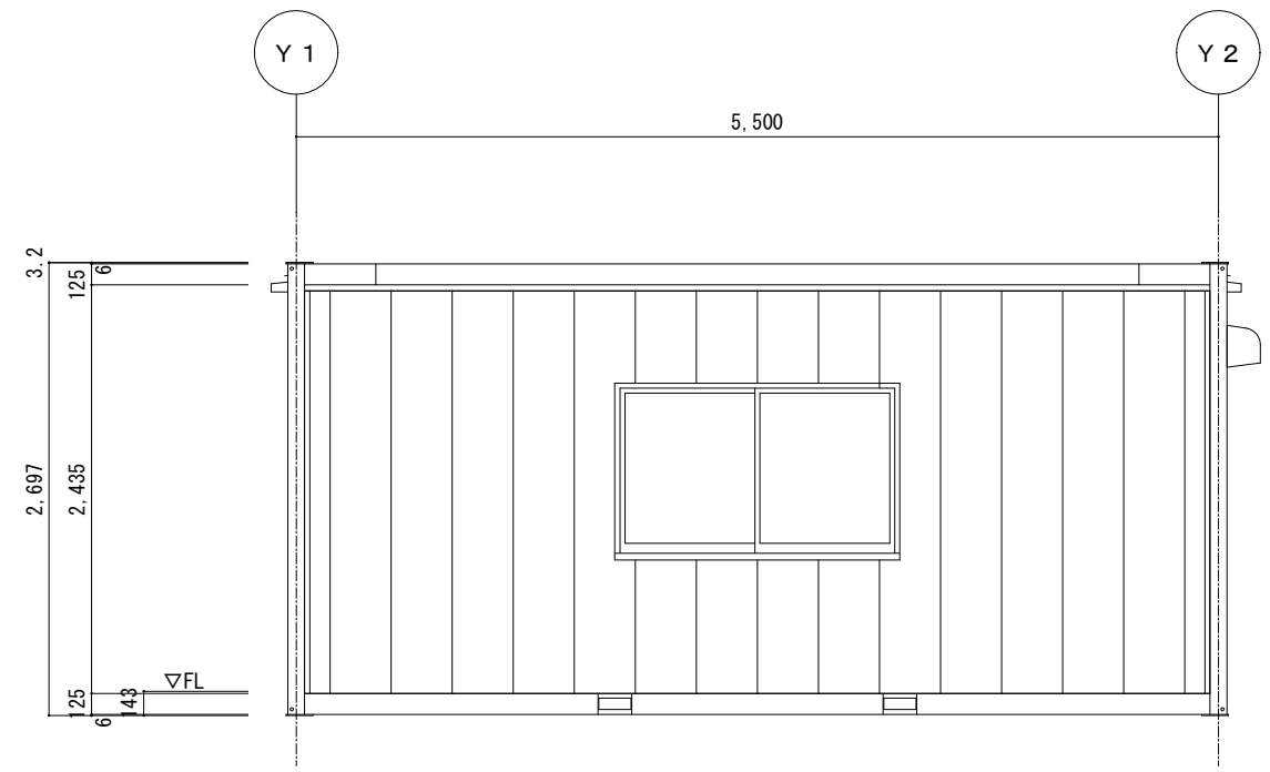
B側立面図 S = 1/50
