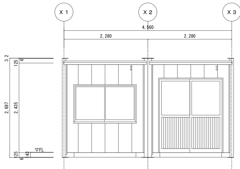
C側立面図 S = 1/50
